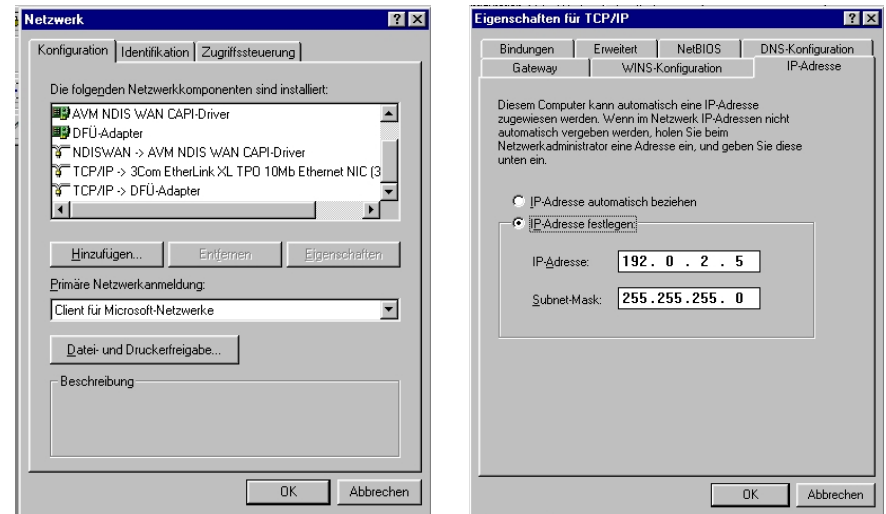
Bild 2 Netzwerkeinstellungen
